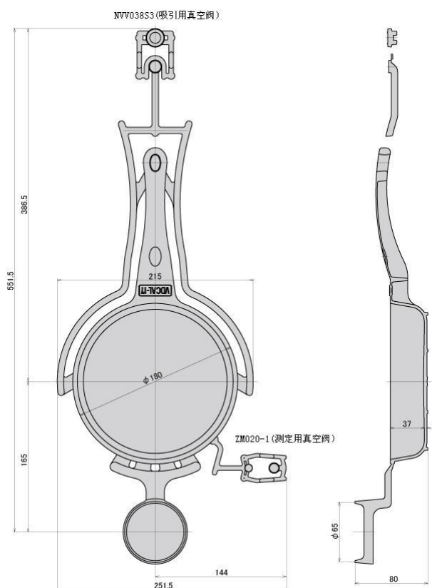
铸造方案规格图
