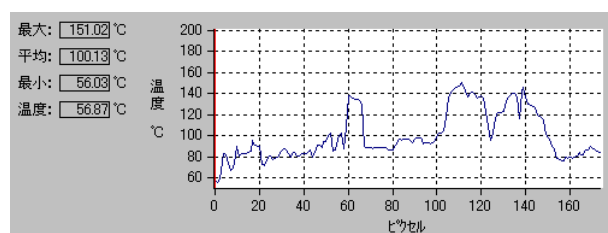
D-2 模具温度
