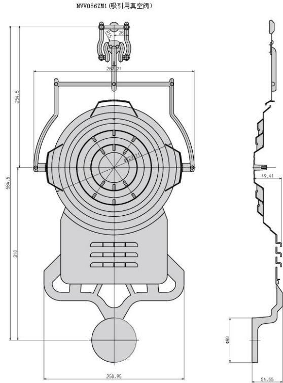
铸造方案规格图
